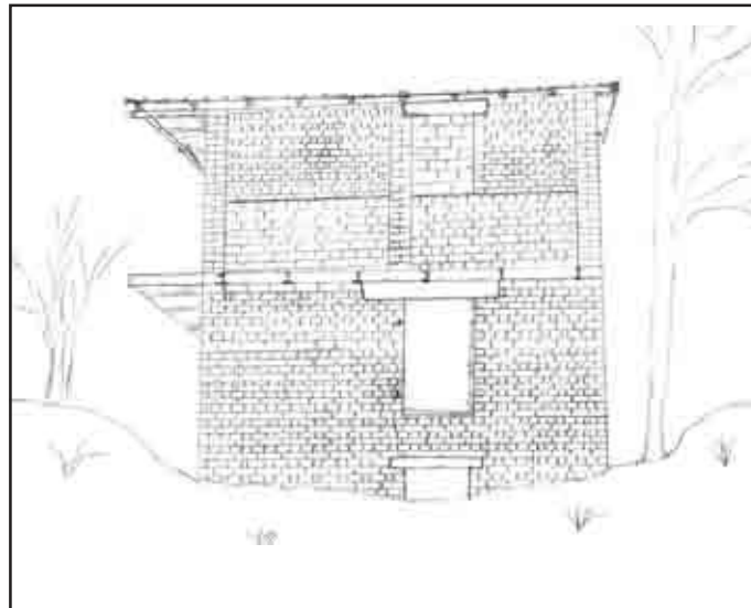
Abb. 7 Skizze der Frontansicht der Brikettwaage nach 1947. Die Skizze zeigt in etwa die neue Frontansicht der Brikettwaage, nachdem der Anbau auf den Fundamenten der Gleiswaage fertig gestellt war. Neben einem Laufweg erkennt man verschiedene Bauabschnitte im Mauerwerk. Quelle: H. W. Breidenbach
